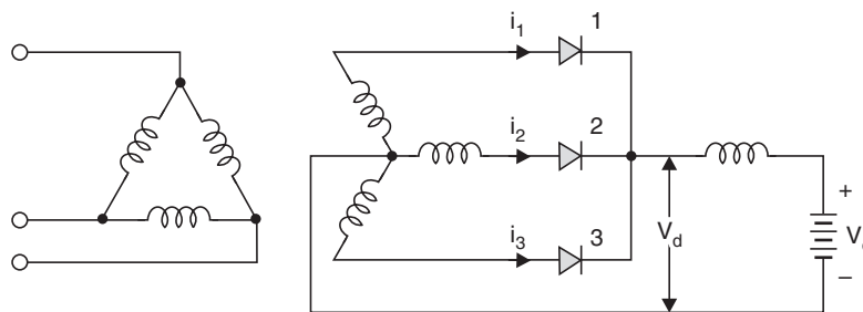
Fig. 5.1 3-phase rectifier.
